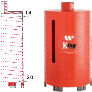
CORPO ESTERNO CONICO CONICAL OUTER BODY CORPS EXTÉRIEUR CONIQUE CUERPO EXTERIOR CÓNICO
